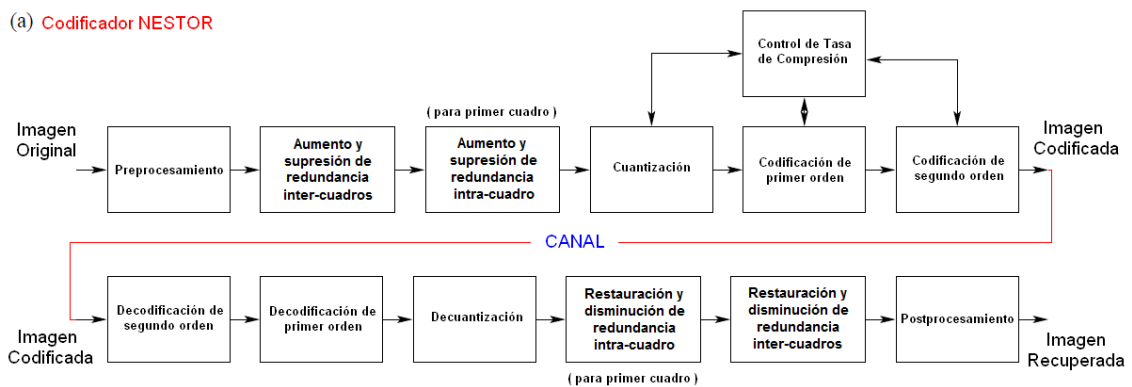
(b) Decodificador NESTOR
