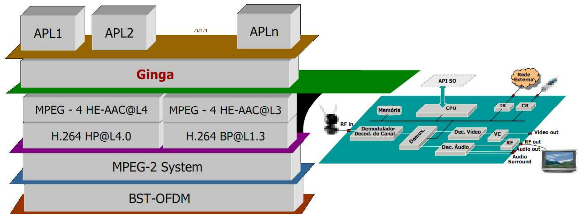
Fig.5: Detalle del set-top-box y las capas desde las aplicaciones interactivas hasta la codificación y modulación.
